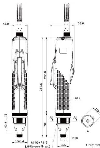
ESL-XTE12/18
