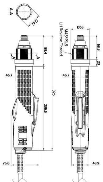
ESL-XTE25
